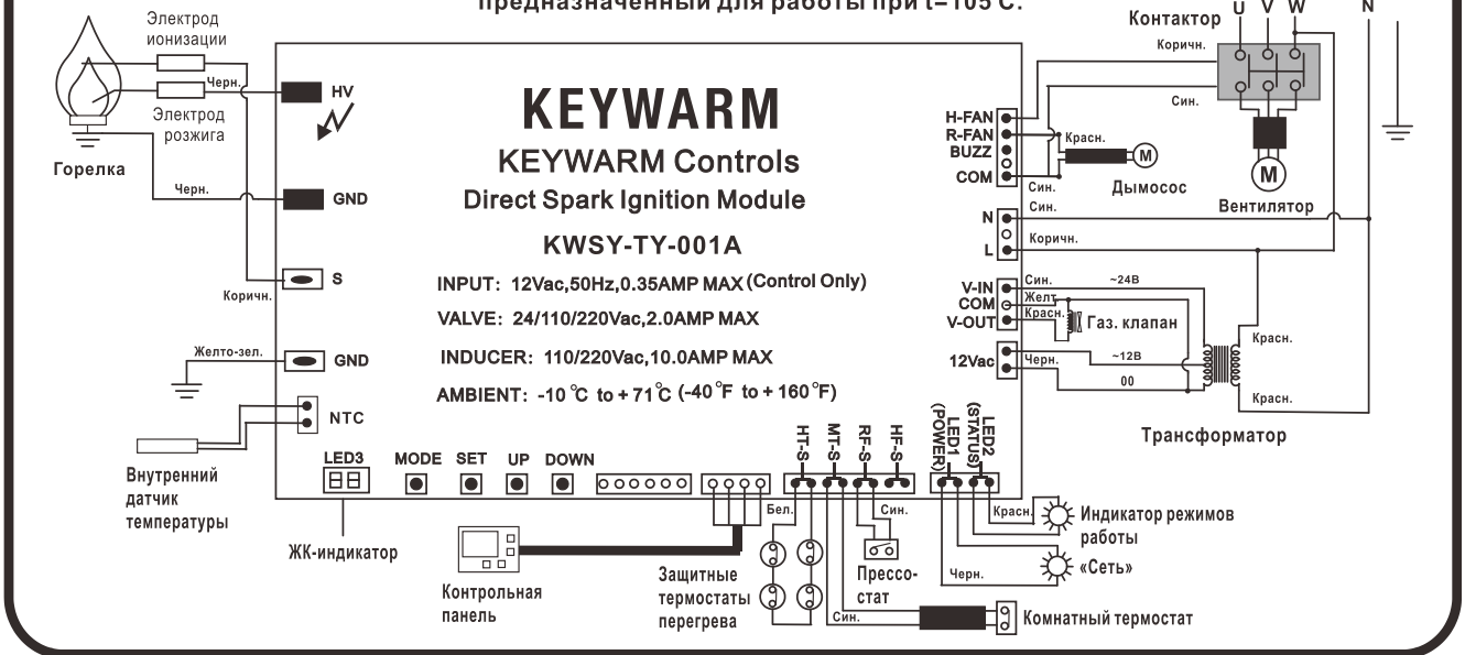
Рис. 4б Схема подключения ~380 В
