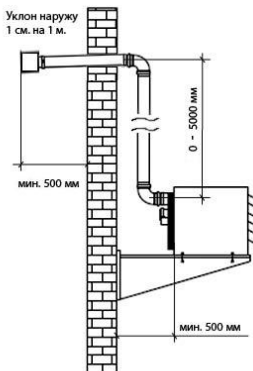
б) вывод дымохода через стену
