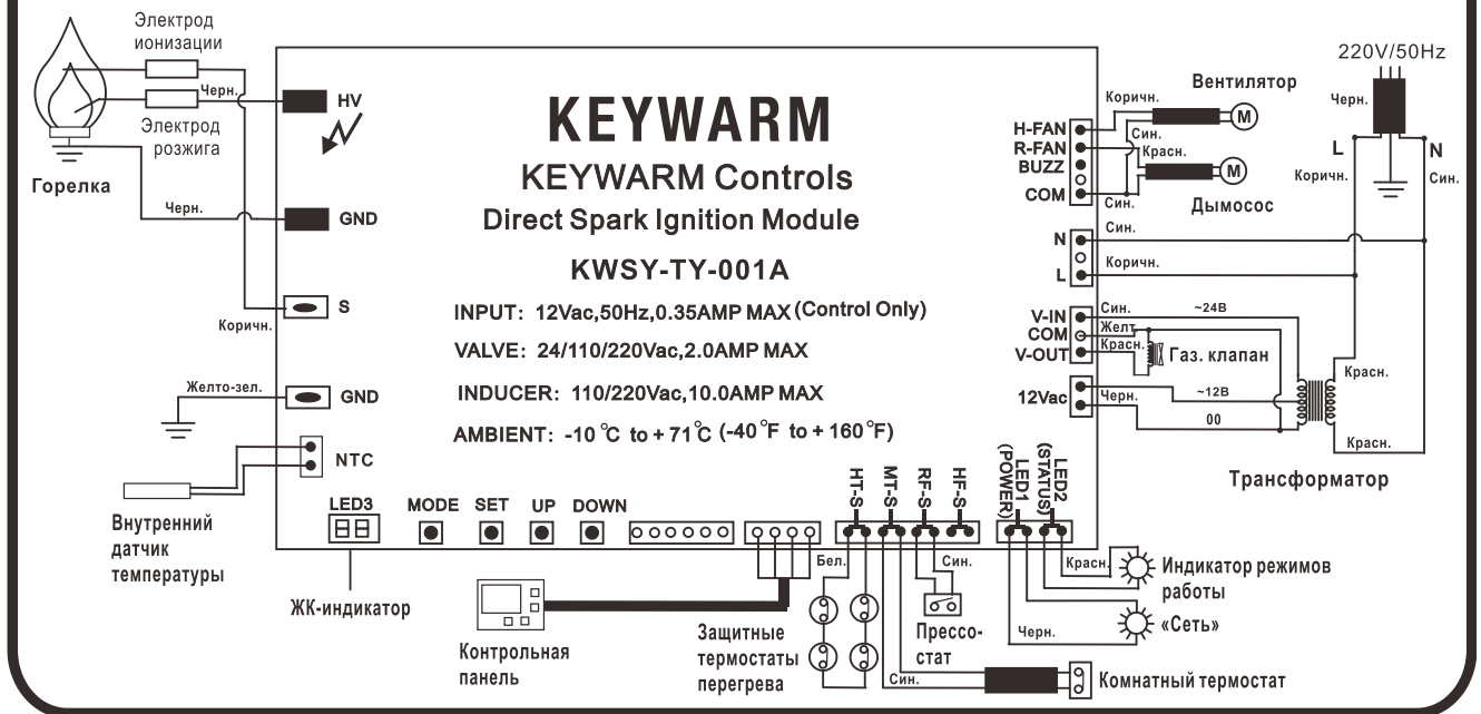
Рис. 4а Схема подключения ~220 В
