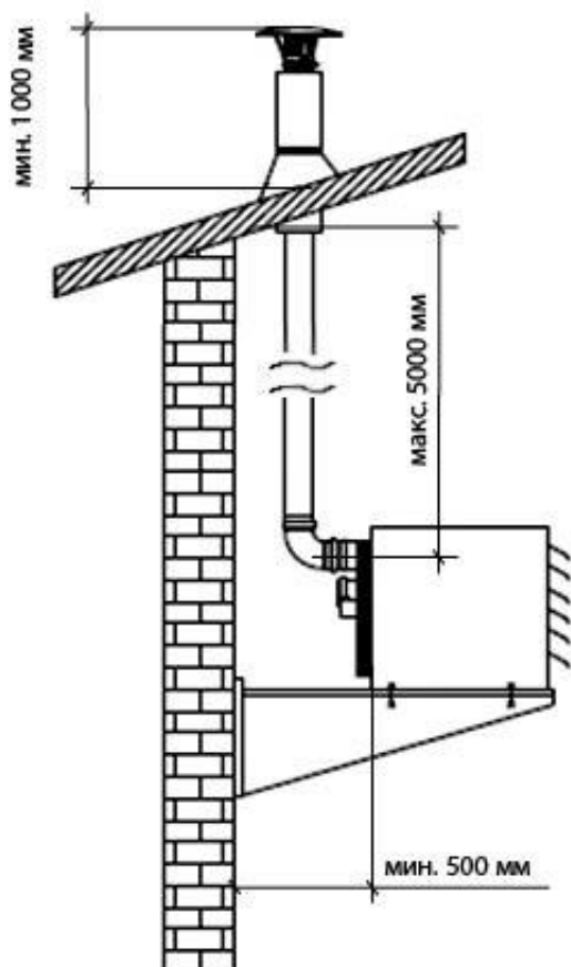
а) вывод дымохода через кровлю
