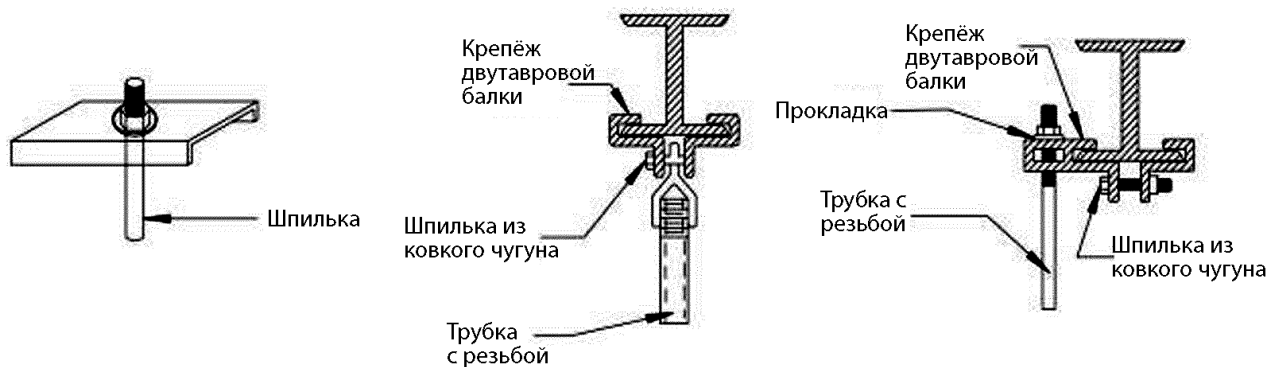
Рис. 3В Крепление нагревателя при монтаже
