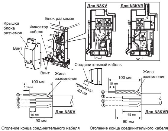
Оголение конца соединительного кабеля
