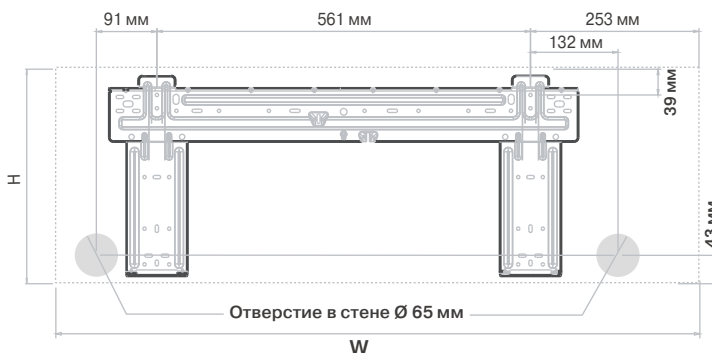
Размеры внутреннего блока (Ш×В): 968 мм x 322 мм
