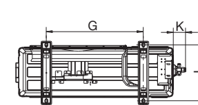
Наружный блок
